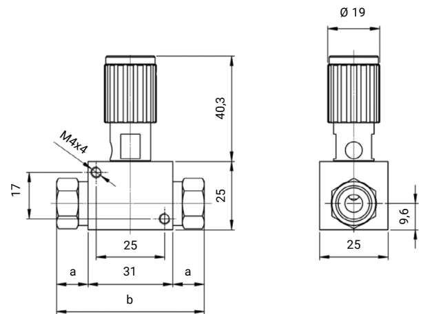
Durchgangsventil - Baugröße klein
